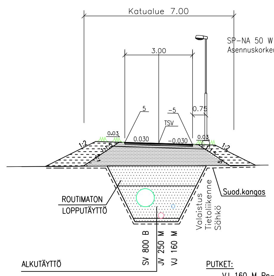
TYYPPIPOIKKILEIKKAUS 1:100 Puistoväylä 1 (pl 10)
