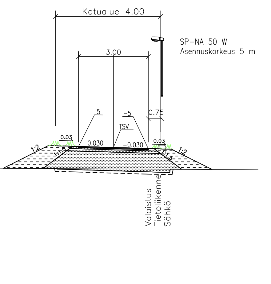
TYYPPIPOIKKILEIKKAUS 1:100 Puistoväylä 3 (pl 10)
