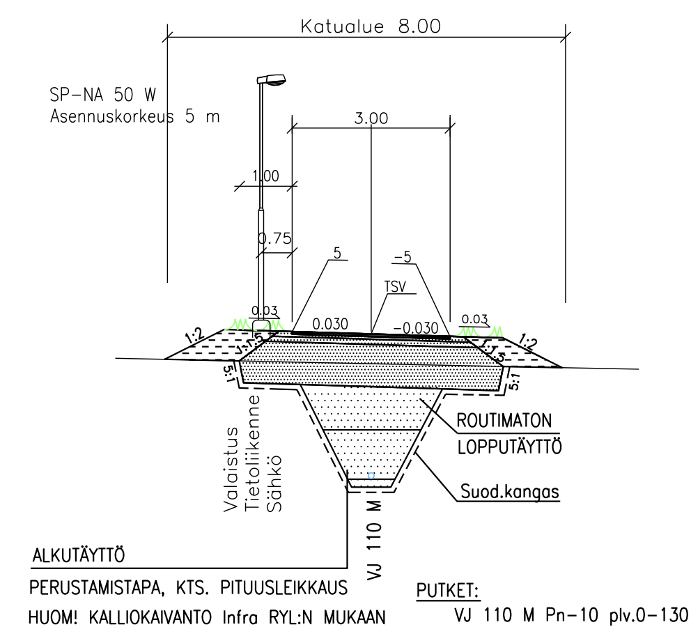
TYYPPIPOIKKILEIKKAUS 1:100 Roihupolku (pl 10)
